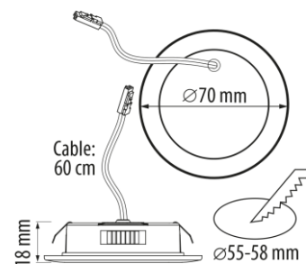
Dimensiones y apertura de montaje.
